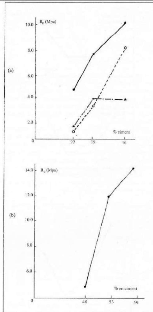
Figure 7 : Résistance à la compression en fonction de la teneur en ciment (a) et (b).
