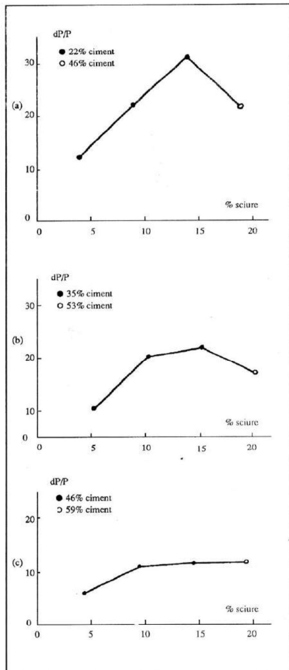
Figure 1 : Pertes de poids en fonction de la teneur en sciure. a) 22% C ; b) 35% C ; c) 46% C.
