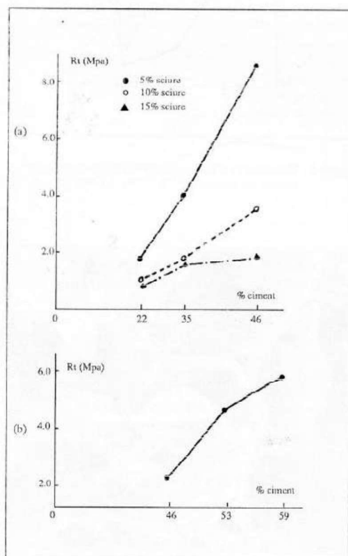
Figure 6 : Résistance à la traction en fonction de la teneur en ciment (a) et (b).
