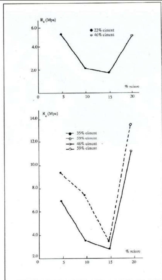
Figure 5 : Résistances à la compression en fonction de la teneur en sciure a) 22% C ; b) 35 % C ; c) 46 % C.
