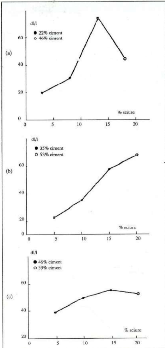
Figure 2 : Variations dimensionnelles en fonction de la teneur en sciure. a) 22% C ; b) 35% C ; c) 46% C.
