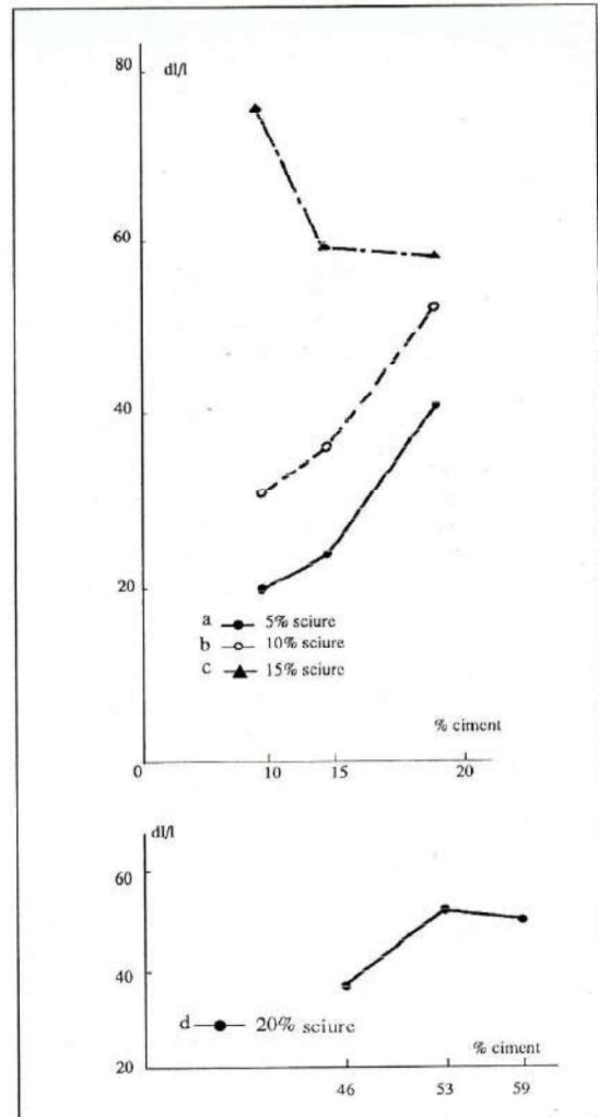
Figure 3 : Variations dimensionnelles en fonction de la teneur en ciment. a) 5% sciure b) 10% sciure ; c) 15% sciure ; d) 20% sciure.
