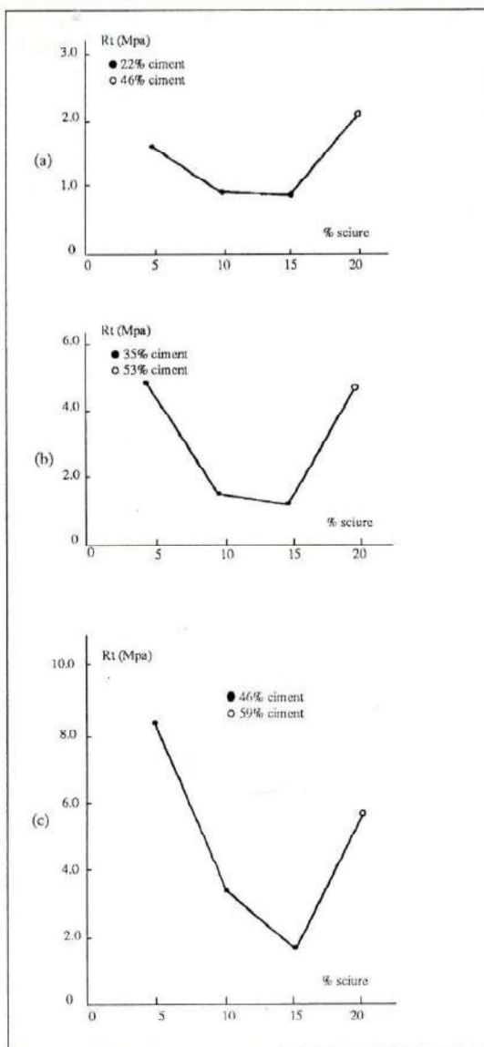
Figure 4 : Résistances à la traction en fonction de la teneur en sciure. a) 22% C ; b) 35% C ; c) 46% C.
