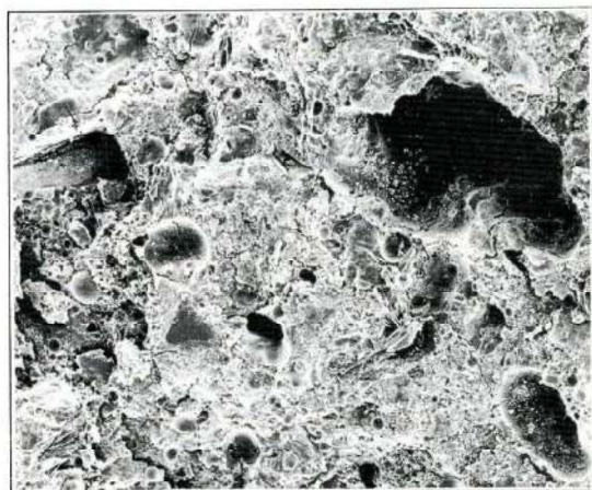
Photo 1 : Texture du mélange. Illustration de la porosité (X 400).
