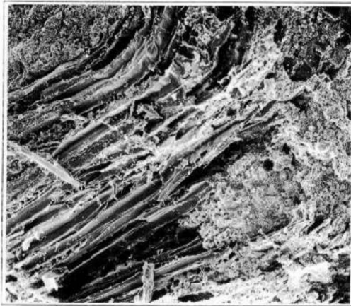
Photo 3 : Pénétration de la pâte de béton dans les vaisseaux de sciure de bois (X 150).
